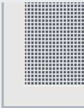
Motiv 413 , Lochblech quadratisch Lüftungsquerschnitt: 45% der Füllungsfläche
