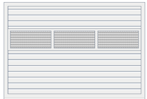
Motiv 480, Lamellenfüllung mit Streckgitter-gefülltem Aluminiumrahmen Lüftungsquerschnitt: 58% der Füllungsfläche pro Rahmen
