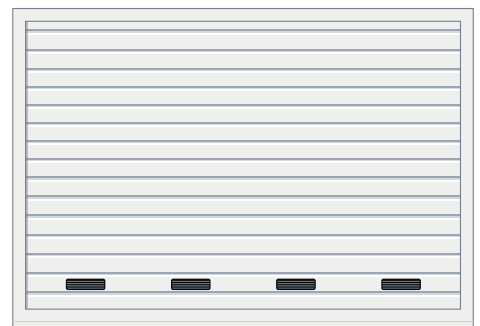
Motiv 480, Lamellenfüllung mit Lüftungsgittern Lüftungsquerschnitt: 40 cm 2 /Gitter
